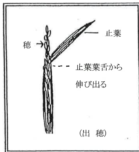
図1 出穂の様子
